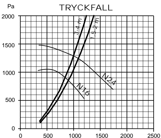
Diagrammet visar variationer i tryckfall och luftflöde för de olika Nederman Original-modellerna i normal arbetsposition.
